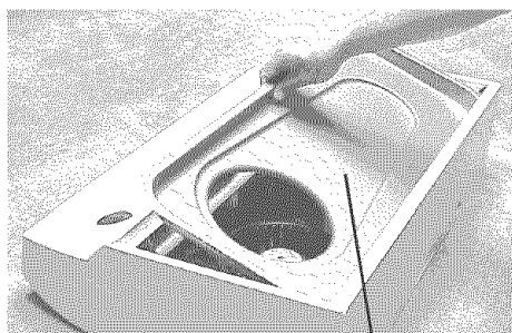
CUBIERTA INFERIOR RECUBIERTA DE TEFLÓN® (Se encuentra fija con 2 tornillos)
