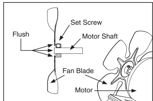
Figure 13. Fan Assembly
