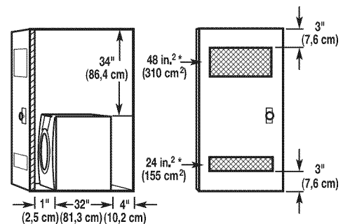
A. Vista lateral – clóset o área confinada B. Puerta del clóset con ventilación
