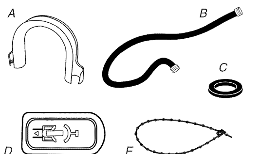
A. Support de tuyau de vidange B. Tuyau d'arrivée d'eau (2) C. Rondelle du tuyau d'arrivée d'eau (4) D. Bouchon du trou du boulon de transport (4) E. Courroie perlée
