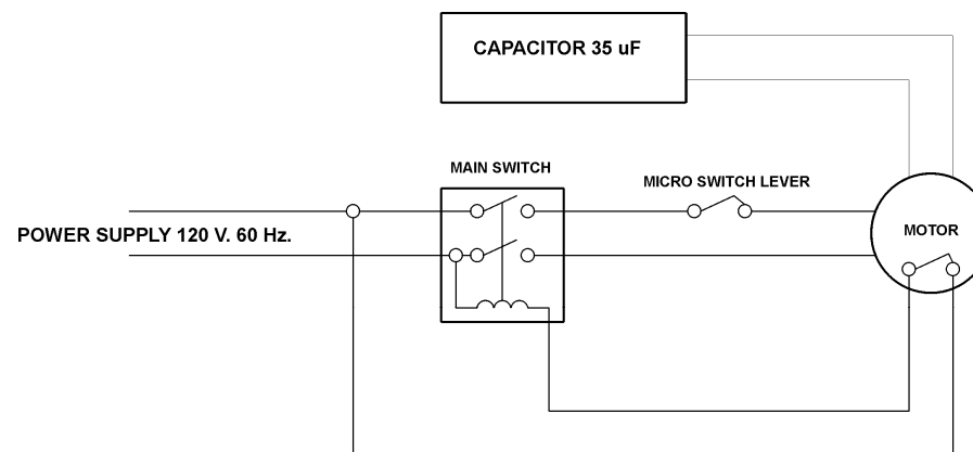
Fig. n°12 - Wiring diagram
