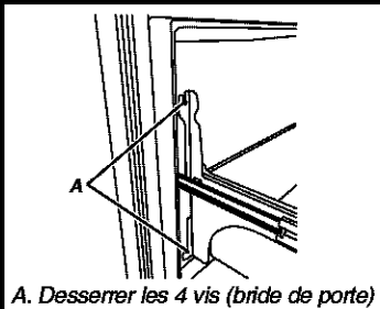
A. Desserer les 4 vis (bride de porte)
