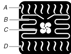
A. Élément de cuisson au grill B. Élément de convection C. Ventilateur de convection D. Élément de cuisson au four
