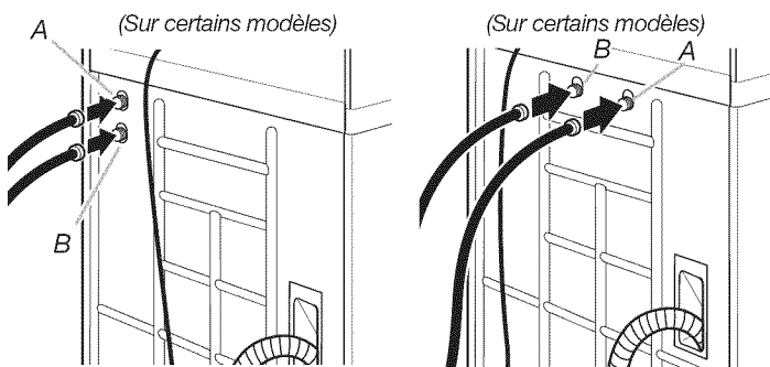
A. Électrovanne d'alimentation — eau froide B. Électrovanne d'alimentation — eau chaude
