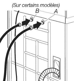
A. Électrovanne d'alimentation — eau froide B. Électrovanne d'alimentation — eau chaude
