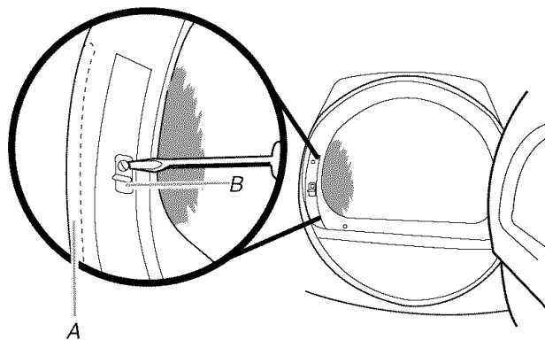
A. Tringle des pitons d'obturation des trous (invisible sous cet angle) B. Gâche de la porte
