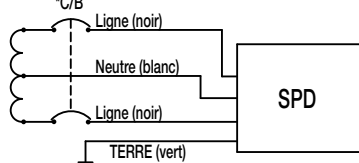
SCHÉMAS DE CÂBLAGE DES SPD DE TYPE 1 ET 2 120/240 VCA MONOPHASÉ
