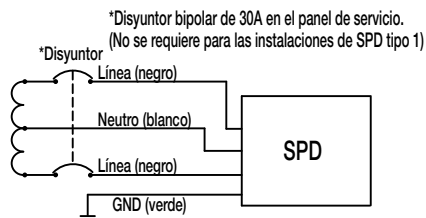
DIAGRAMA DE CABLEADO DE SPD TIPO 1 Y 2 MONOFÁSICO DE 120-240 V CA
