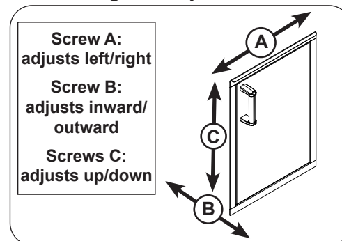
Fig. 4-3 Adjust door
