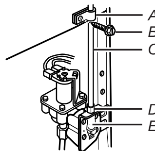
A. Bride du tube B. Vis de bride du tube C. Tube en cuivre D. Écrou de compression E. Valve d'entrée d'eau
