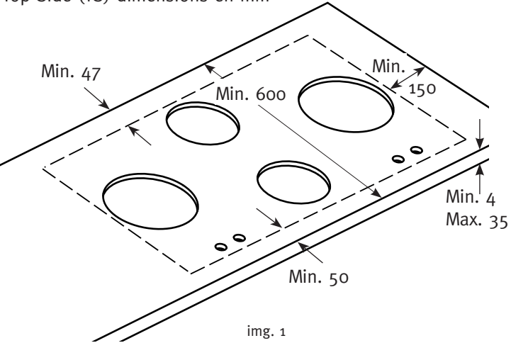
Top Side (TS) dimensions en mm
