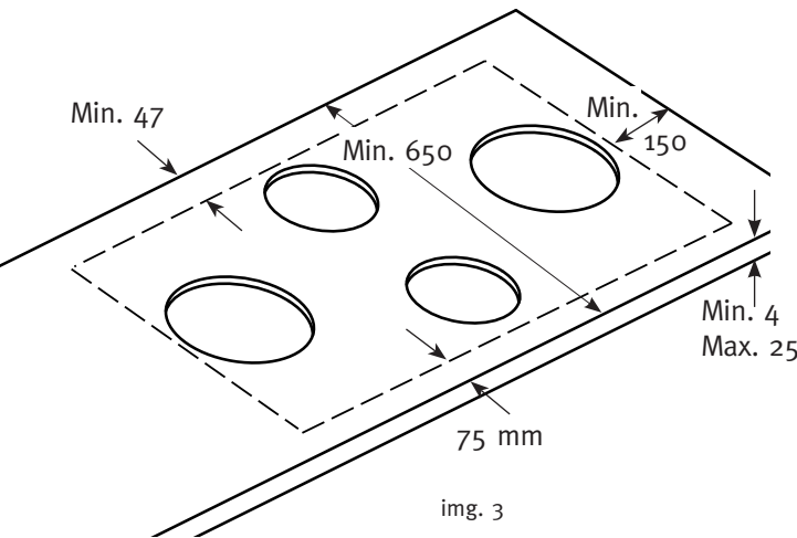
Front Side (FS) dimensions en mm
