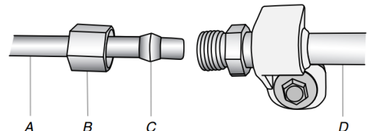
A. Canalisation d'eau du domicile B. Écrou (à acheter) C. Virole (à acheter) D. Tuyau d'eau du réfrigérateur
