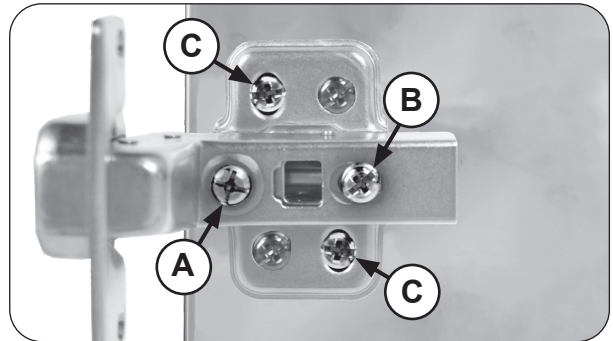
Fig. 14-3 Door hinge detail
