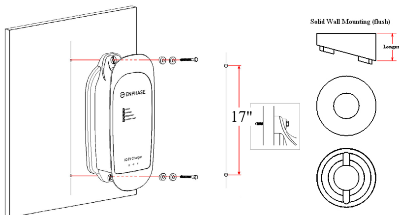
Figure 9 : Montage de l'EVSE sur une paroi pleine
