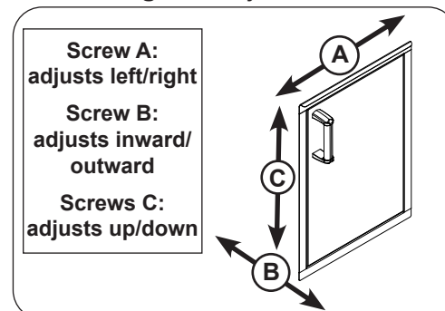
Fig. 4-3 Adjust door
