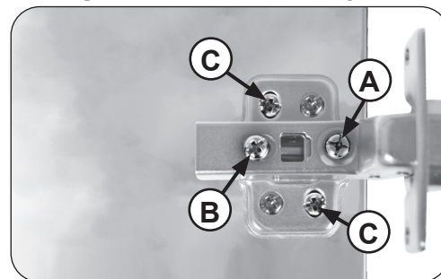
Fig. 4-2 Adjust door
