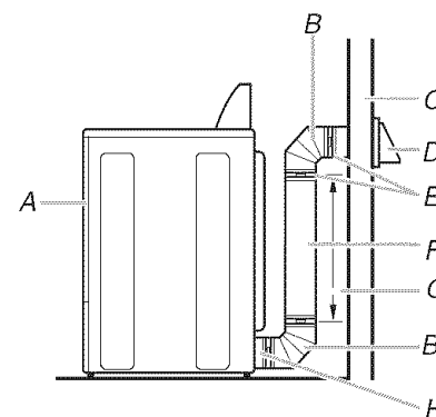
F. Conduit métallique rigide ou souple G. Longueur de conduit nécessaire pour raccorder les coudes H. Bouche de décharge
