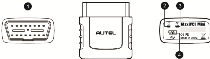
Figure 2-4 MaxiVCI Mini Views
