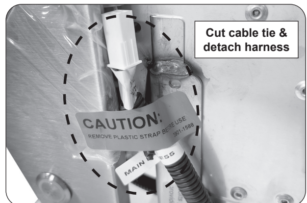
Fig. 28-3 Cut cable-tie
