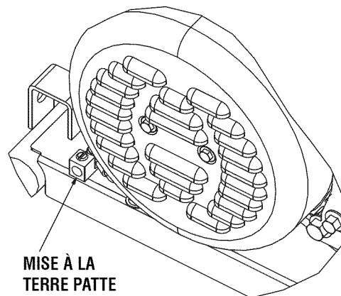
Schéma 8 - Mise à la terre du générateur
