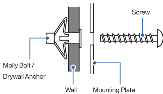
Hollow Drywall
