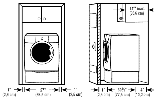
A. Encastrément B. Vue latérale - placard ou endroit exigu
