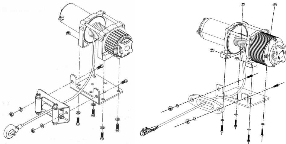
Figur 7 - vinschmontering
