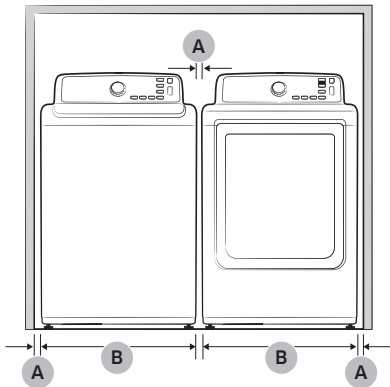
Área empotrada
