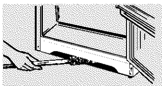
Limpieza de las espirales del condensador.
