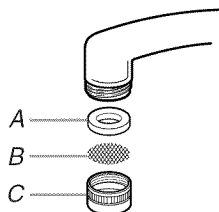
A. Arandela B. Filtro C. Portafiltro o aereador
