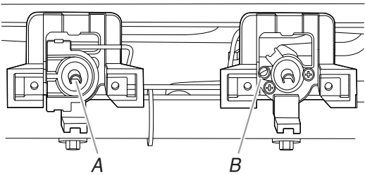
A. Tornillo de ajuste bajo-reducción para la válvula de aluminio a través del centro del vástago B. Tornillo de ajuste bajo-reducción para la válvula de cobre
