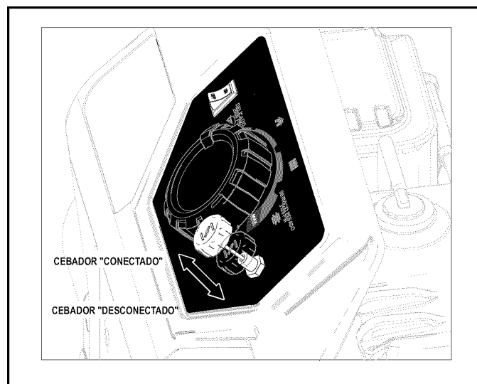
Figura 5-4. Perilla del cebador
