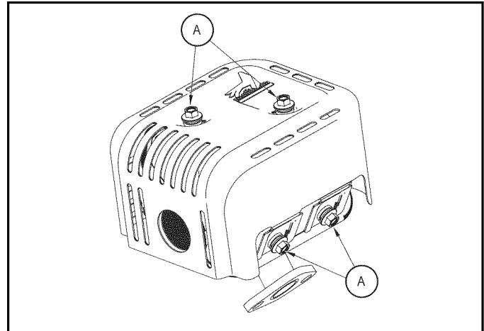
Figura 6-10. Retiro del protector de calor
