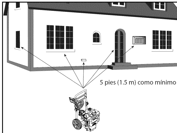
Figura 5-1. Separación de edificios
