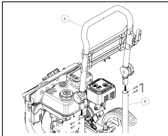
Figura 4-3. Fijación del asa en la unidad
