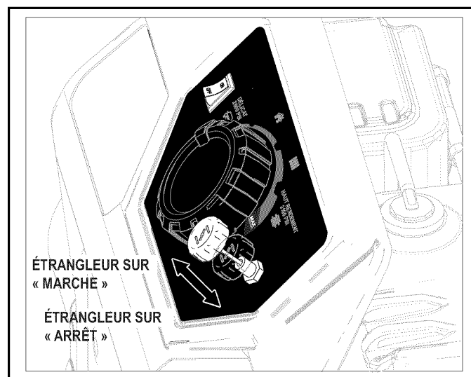
Figure 5-4. Bouton de l'étrangleur
