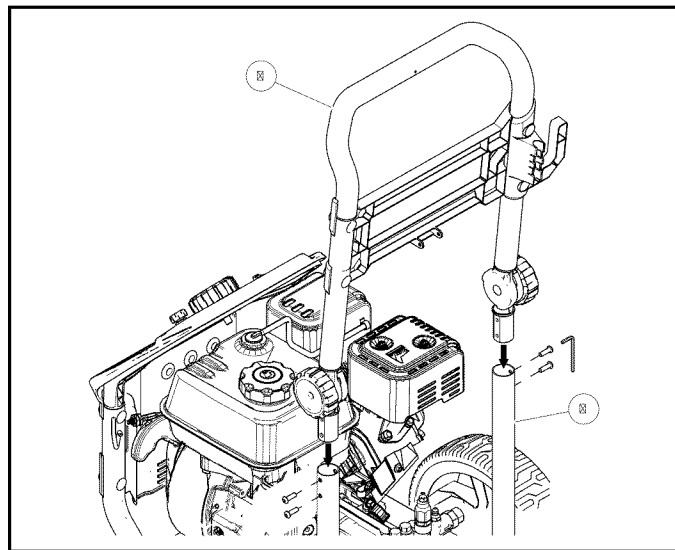
Figure 4-3. Attacher la poignée à l'appareil
