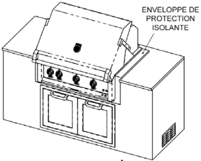
INSTALLATION EN ÎLE TYPIQUE AVEC ENVELOPPE DE PROTECTION ISOLANTE (GRIL 36 po REPRÉSENTÉ)
