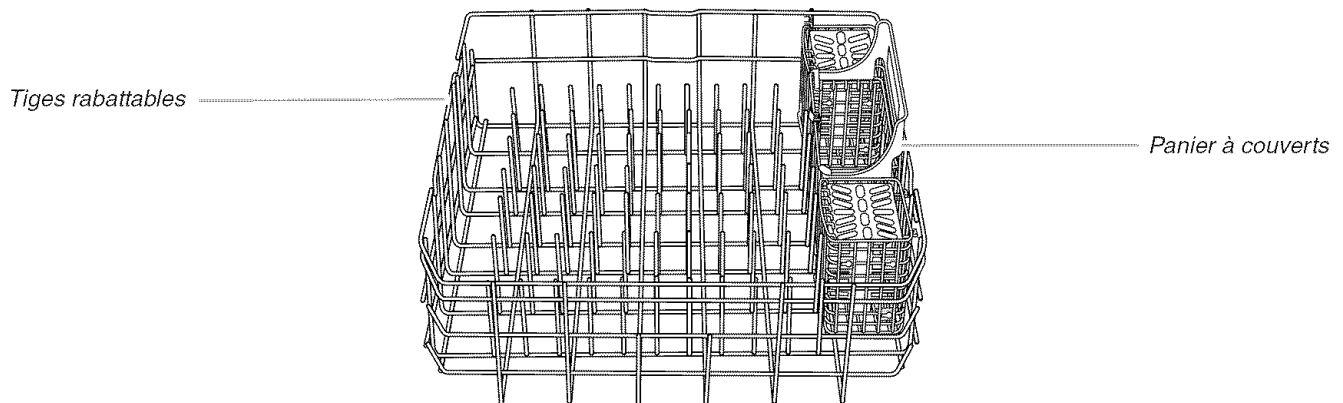
PANIER INFÉRIEUR
