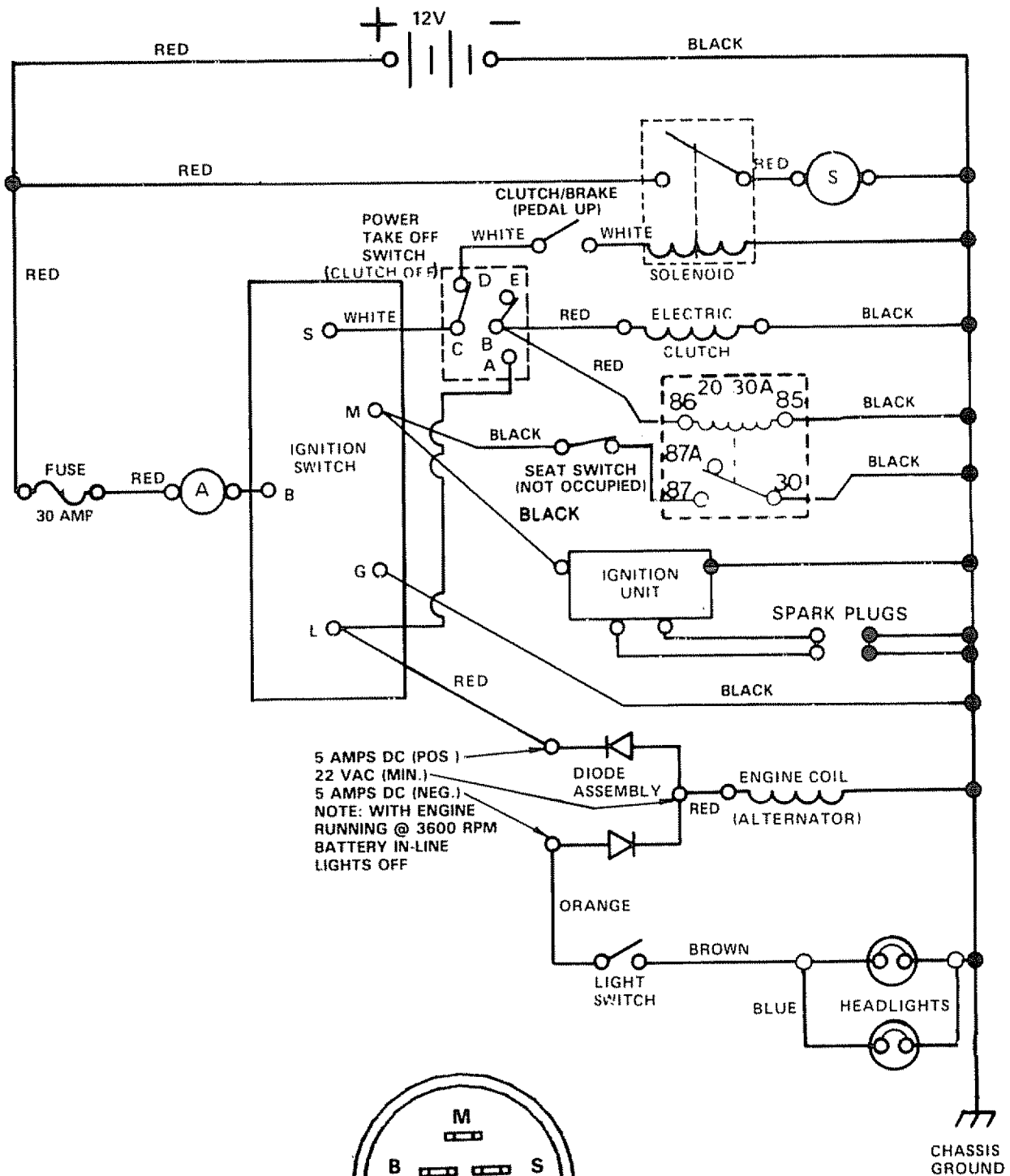
PTO SWITCH
