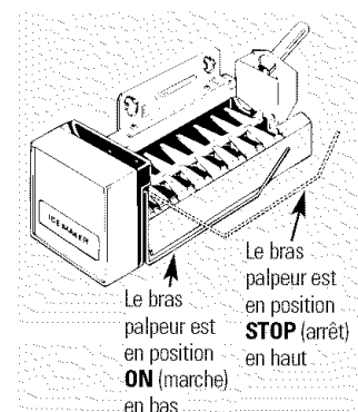
Modèle à bras palpeur
