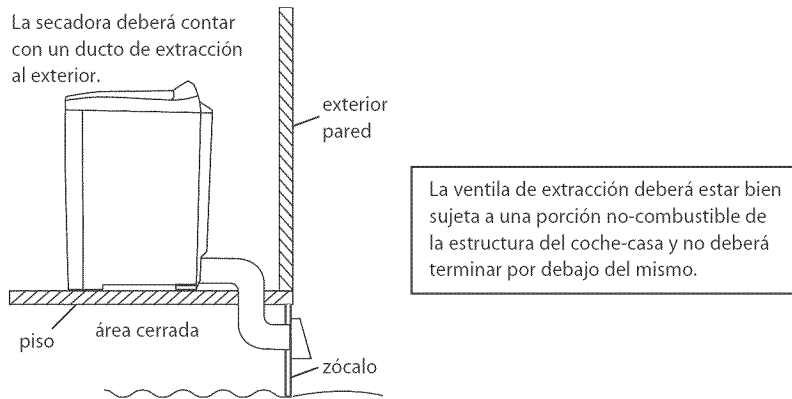
Dibujo 8 Ventilación exterior
