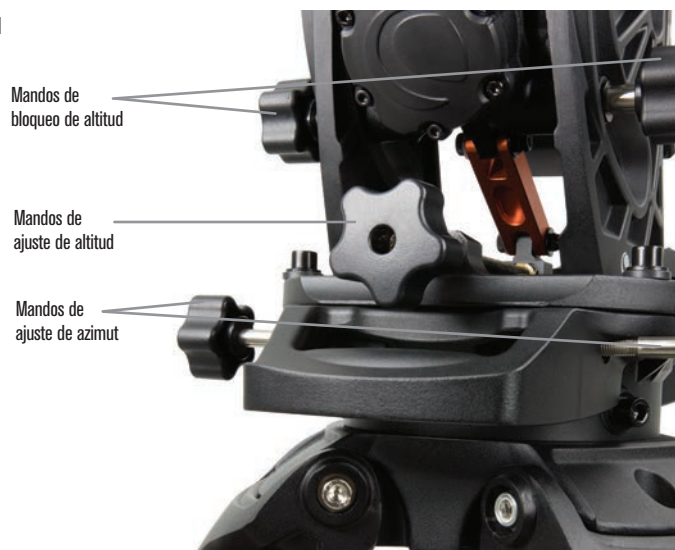
Figura 8 Regulación de alineación polar
