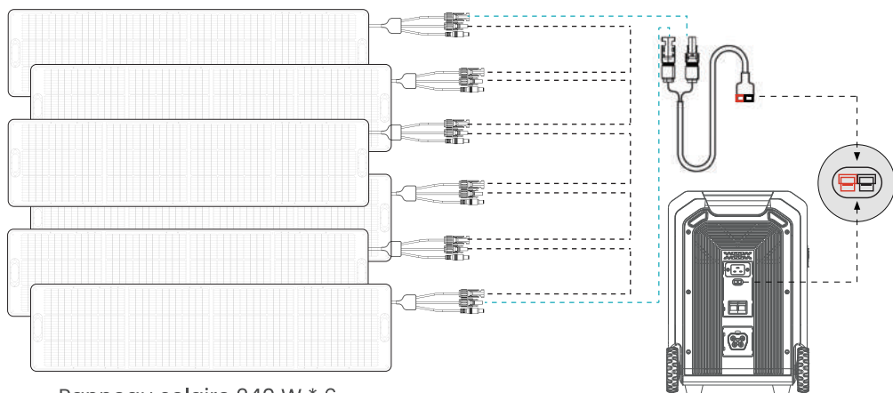
Panneau solaire 240 W * 6
