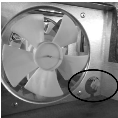
Revised Fan Shroud
