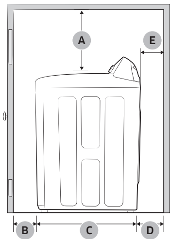
Vista lateral - gabinete o área reducida
