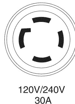
Schéma 7 - Prise de 120/240 Volts CA, 30 Amp
