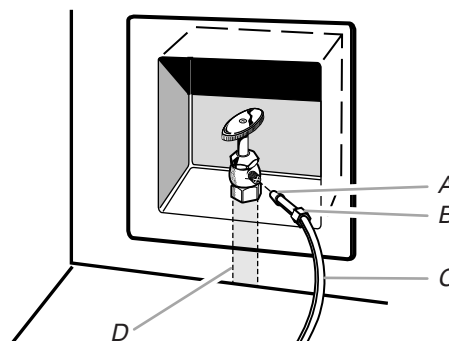
A. Bague B. Écrou C. Tube en cuivre (jusqu'au réfrigérateur) D. Canalisation d'alimentation en eau du domicile (1/2" minimum)
