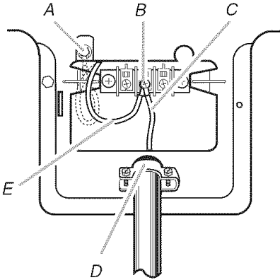
A. Tornillo conductor de tierra externo – La línea punteada ilustra la posición del hilo de tierra NEUTRO antes de moverlo al tornillo central de color plateado del bloque de terminal. B. Tornillo central de color plateado del bloque de terminal C. Hilo neutro (hilo blanco o central) D. Protector de cables de 3/4" (1,9 cm), que esté en la lista de UL E. Hilo neutro de puesta a tierra
