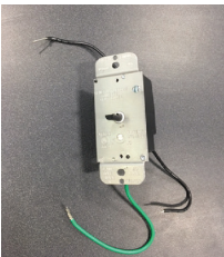
BC10 Variable Wall Rheostat
