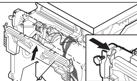
Ensamblaje de la bandeja de goteo
