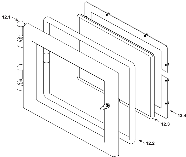
#12 Door Assembly
