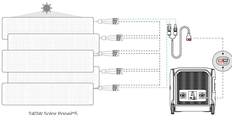
240W Solar Panel*5
