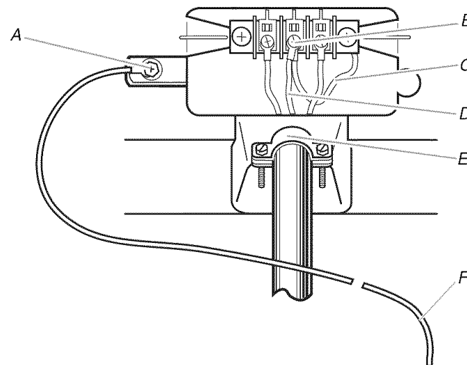
A. Tornillo conductor de tierra externo B. Tornillo central de color plateado del bloque de terminal C. Hilo neutro de puesta a tierra D. Hilo neutro (hilo blanco o central) E. Protector de cables de \frac{3}{4} " (1,9 cm), que esté en la lista de UL F. Camino de puesta a tierra determinado por un electricista capacitado
