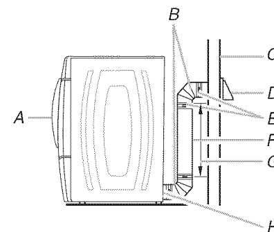
A. Sécheuse B. Coude C. Mur D. Clapet de décharge E. Brides
