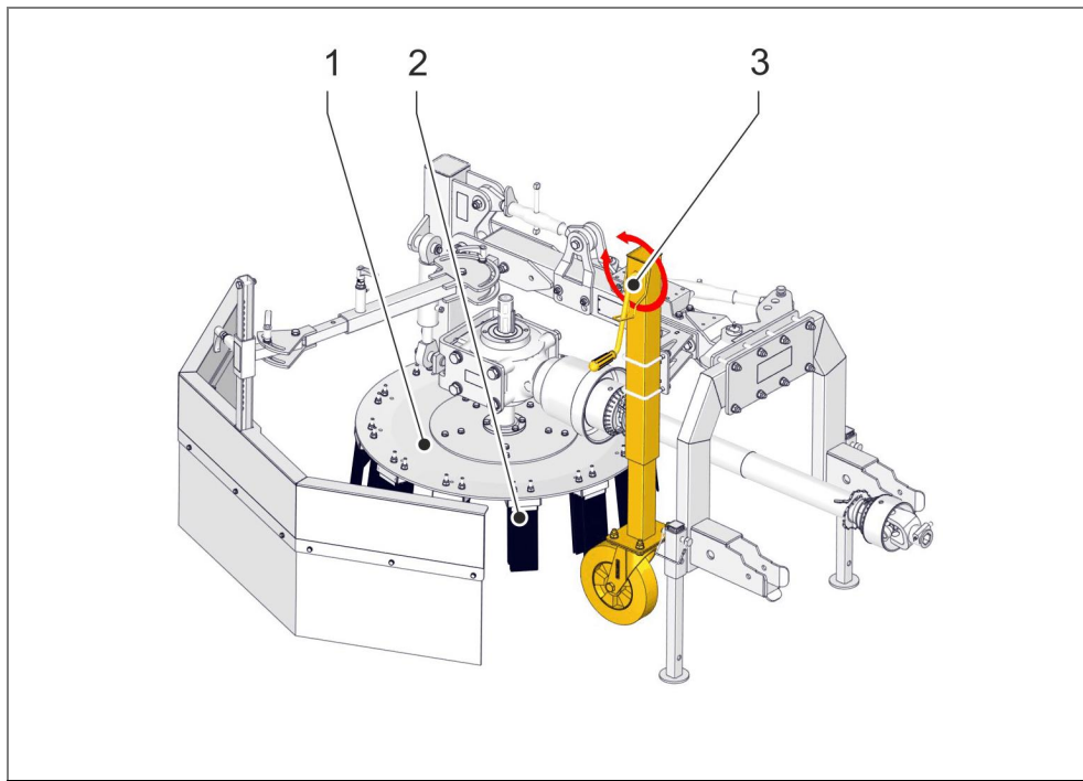
Fig. 4 : réglage du porte-brosse
