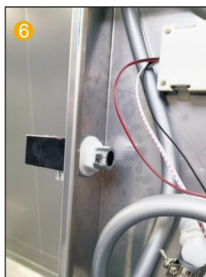
6 Insérez la buse de pulvérisation manuelle dans le panneau et installez le joint.
