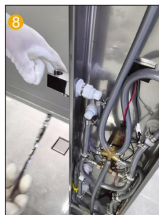
8 Connectez le connecteur de sortie d'eau à la main connecteur de siège de pulvérisation.
