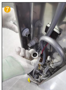
7 Mettre le caoutchouc à 4 voies dans le connecteur du siège avec douche à main.
