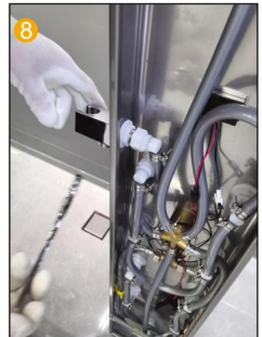
8 Schließen Sie den Wasserauslassanschluss an die Hand Sprühitzanschluss.
