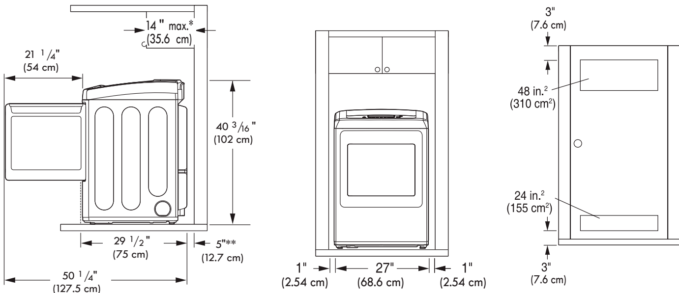
Closet Door Vent Requirements
