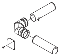
Kit de ventilación lateral* N.º de kit: 26-49670
