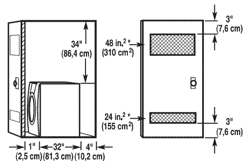
A. Vista lateral - clóset o área confinada B. Puerta del clóset con ventilación
