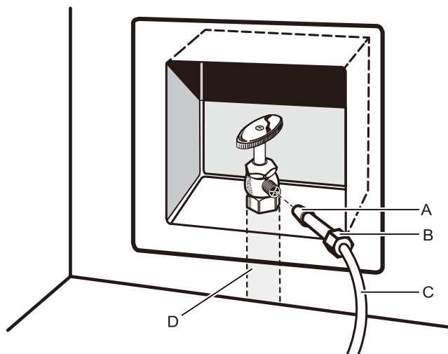
A. Manchon B. Écrou C. Tube en cuivre (vers le réfrigérateur) D. Ligne d'alimentation domestique
