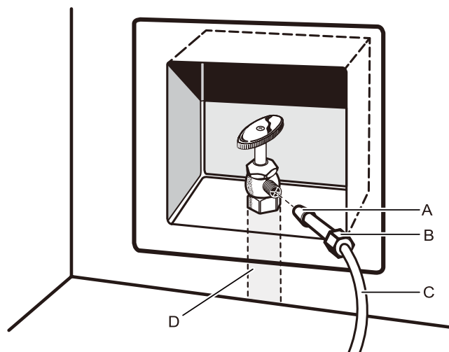
A. Manguito C. Tubería de cobre (al frigorífico) B. Tuerca D. Línea de suministro doméstico
